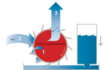
Sistema di umidificazione
