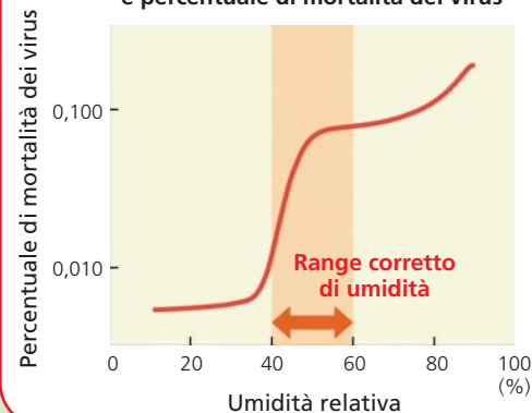
Rapporto tra umidità relativa e percentuale di mortalità dei virus
